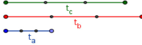
شكل 8: تثليث متوسطات المثلث
